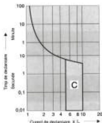
Caracteristica de declansare C
